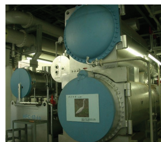
下水熱利用ヒートポンプ
