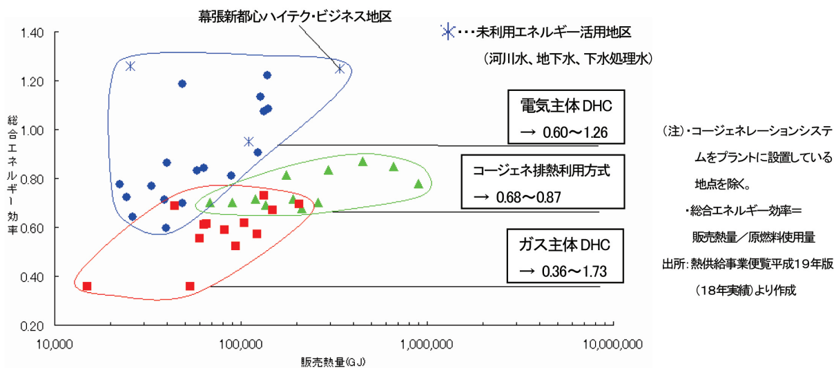
当社管内地域熱供給（DHC）地区の総合エネルギー効率
